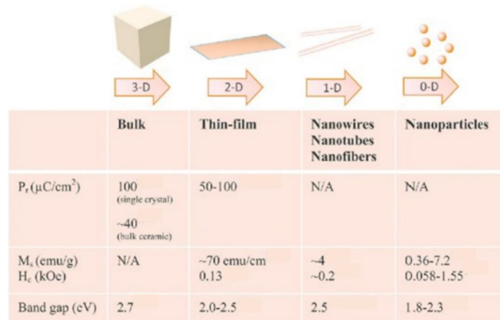
Gambar 1. Bismuth ferrite dengan berbagai struktur dimensi dan sifat-sifatnya yang dihasilkan [33]
