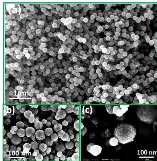
Gambar 4. (a,b) SEM dan (c) FESEM dari mikrosfer kluster \text{Bi}_{25}\text{FeO}_{40} [24]
