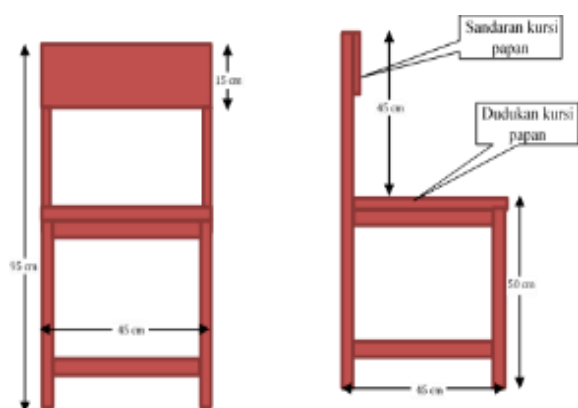
Gambar 1. Dimensi kursi kayu yg akan dibuat atau direkondisi
