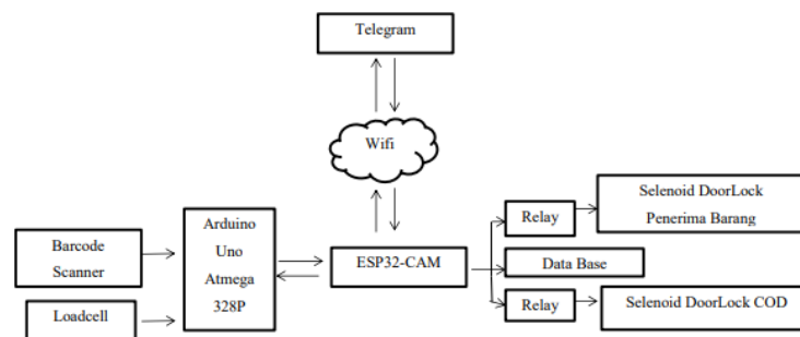
Gambar 1. Diagram Blok Perancangan Perangkat Keras
